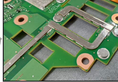
大電流配線 High current on the pattern
