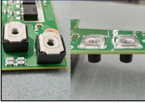
金属粉対策 Contamination prevention
