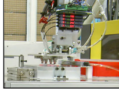
除電・防塵のアップ Static elimination & dust proof
