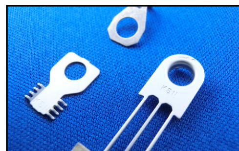
アース端子 Earth(GND) terminal
